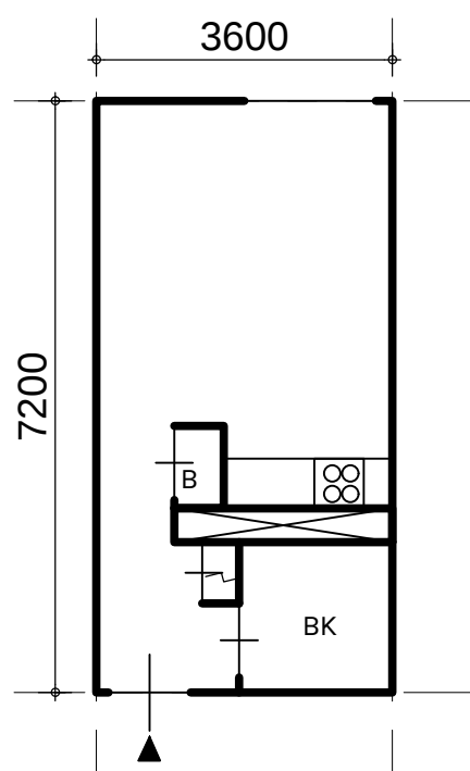
Festing eenkamerwoning
